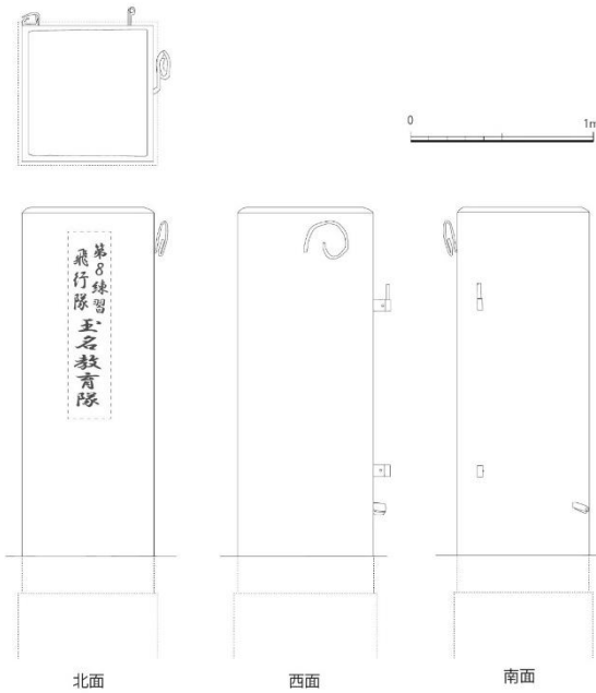
大浜飛行場正門東側門柱実測図
