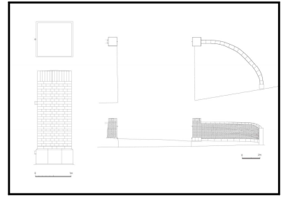
十三聯隊正門の測量図
